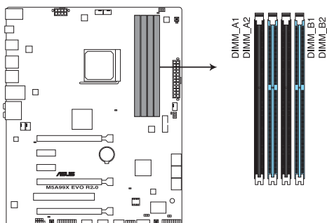
Interfaces de connexion pour modules mémoire DDR3 de la M5A99X EVO R2.0
