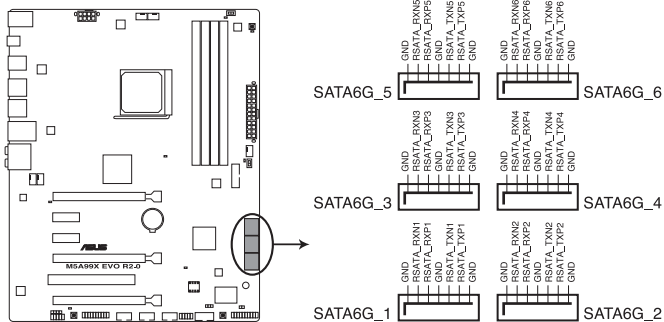
Connecteurs SATA 6.0Gbs de la M5A99X EVO R2.0
