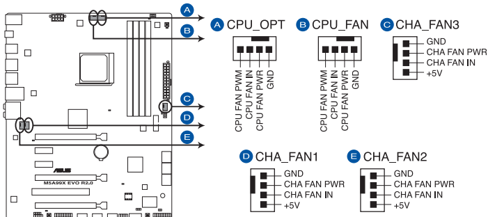
Connecteurs de ventilation de la M5A99X EVO R2.0
