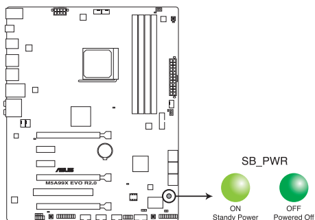
LED d'alimentation de la M5A99X EVO R2.0
