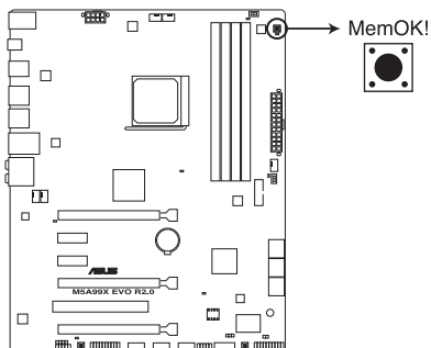
Bouton MemOK! de la M5A99X EVO R2.0
