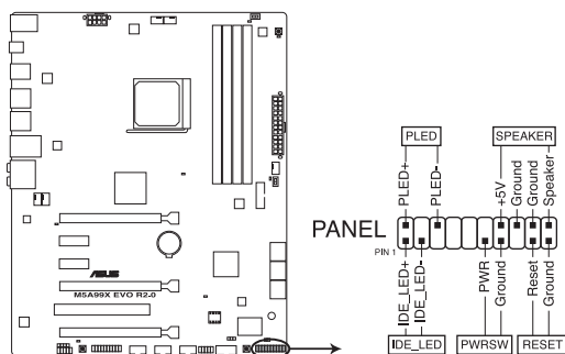
Connecteur panneau système de la M5A99X EVO R2.0
