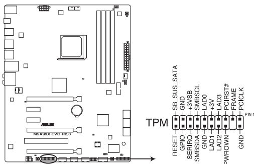
Connecteur TPM de la M5A99X EVO R2.0
