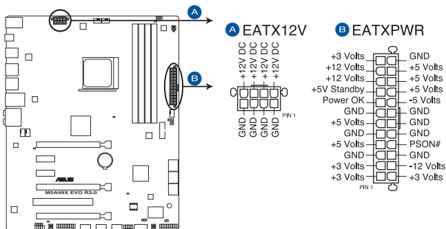
Connecteurs d'alimentation de la M5A99X EVO R2.0
