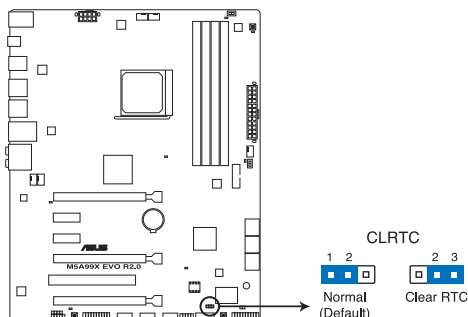
Jumper d'effacement de la mémoire RTC de la M5A99X EVO R2.0
