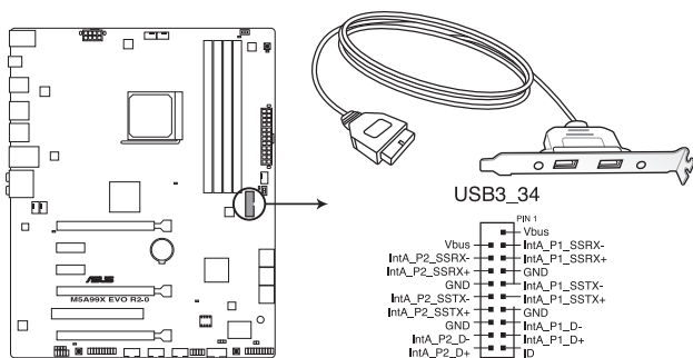
Connecteur USB 3.0 de la M5A99X EVO R2.0
