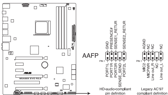
Connecteur audio pour panneau avant de la M5A99X EVO R2.0
