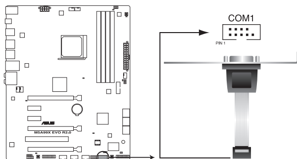
Connecteur COM de la M5A99X EVO R2.0
