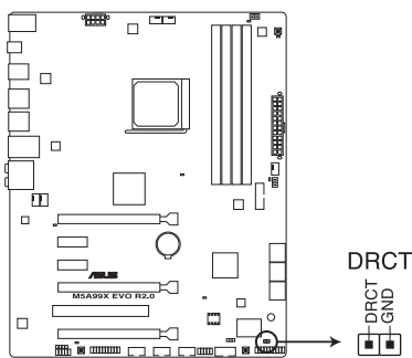
Connecteur DirectKey de la M5A99X EVO R2.0
