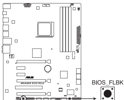
Bouton BIOS Flashback de la M5A99X EVO R2.0
