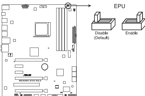
Interrupteur EPU de la M5A99X EVO R2.0
