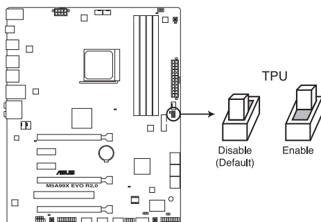
Interrupteur TPU de la M5A99X EVO R2.0
