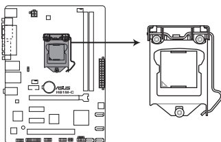
Interface de connexion LGA1150 de la H81M-C
