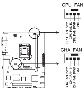
Connecteurs de ventilation de la H81M-C
