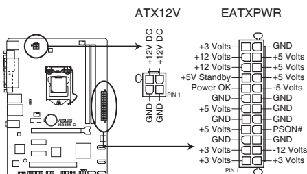
Connecteurs d'alimentation de la H81M-C
