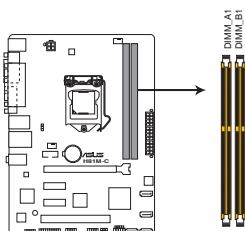
Interfaces de connexion pour modules mémoire DDR3 de la H81M-C
