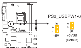
Jumper de mise en route via clavier et USB de la H81M-C
