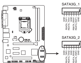
Connecteurs SATA 6.0Gbs de la H81M-C
