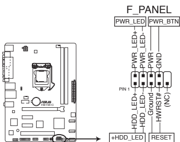
Connecteur panneau système de la H81M-C
