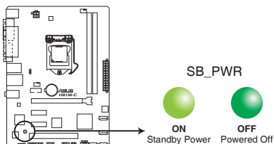
Voyant d'alimentation de la H81M-C
