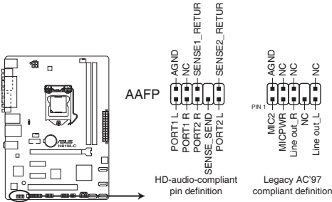
Connecteur audio pour panneau avant de la H81M-C
