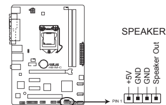
Connecteur pour haut-parleur d'alerte système de la H81M-C
