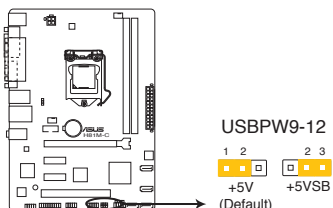
Jumper de mise en route via USB de la H81M-C
