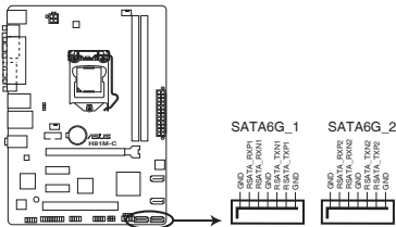
Connecteurs SATA 6.0Gbps de la H81M-C
