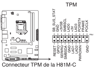
Connecteur TPM de la H81M-C
