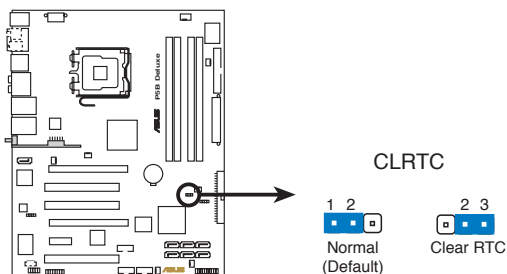
Clear RTC RAM de la P5B Deluxe
