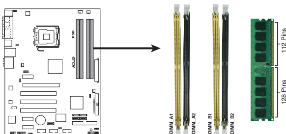
Sockets DIMM DDR2 de la P5B Deluxe
