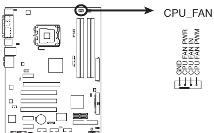
Connecteur CPU_FAN de la P5B Deluxe
