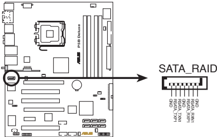
Connecteur RAID SATA de la P5B Deluxe
