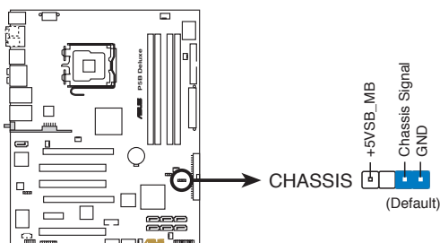
Connecteur Châssis intrusion de la P5B Deluxe
