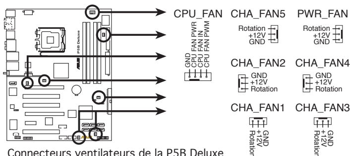
Connecteurs ventilateurs de la P5B Deluxe
