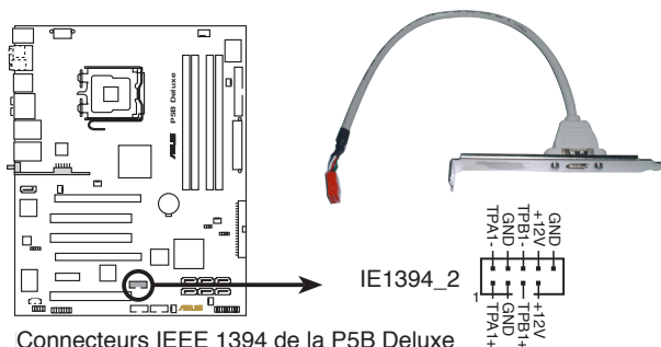
Connecteurs IEEE 1394 de la P5B Deluxe
