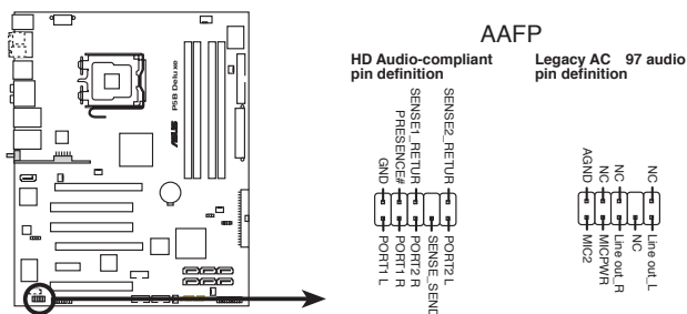
Connecteur Front panel audio de la P5B Deluxe
