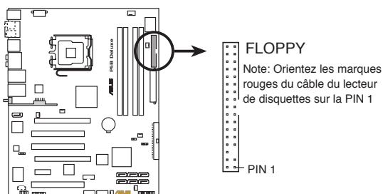
Connecteur pour lecteur de disquettes de la P5B Deluxe
