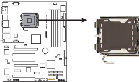
Socket 775 du CPU de la P5B Deluxe
