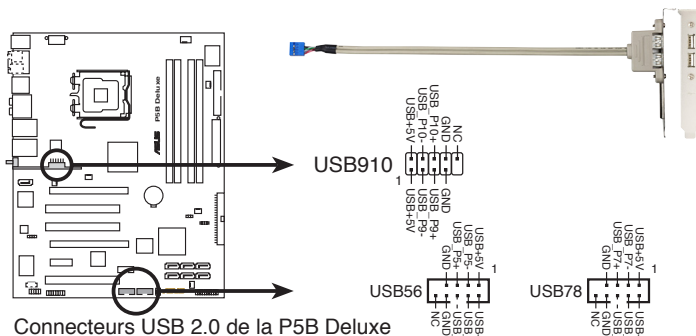
Connecteurs USB 2.0 de la P5B Deluxe
