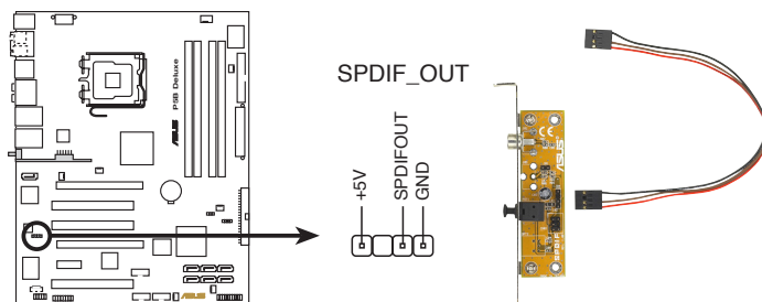
Connecteur audio numérique de la PSB Deluxe
