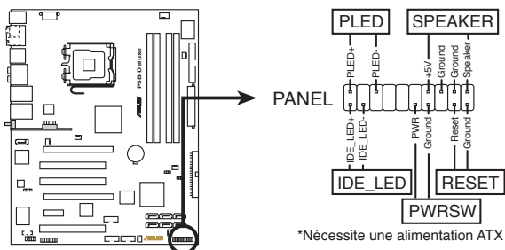
Connecteur System panel de la P5B Deluxe
