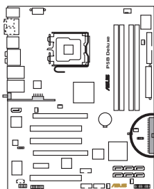
Connecteur IDE de la P5B Deluxe
